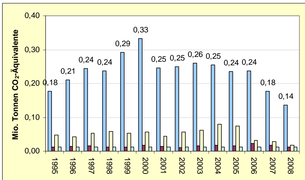
Abbildung 8.1: Emissionen fluoriertes Gase aus der Halbleiterindustrie (von links: FKW, HFKW, SF 6 ) und aus der Leiterplatten(LP)fertigung (rechte Säule) in Deutschland in Mio. t CO 2 -Äquivalente. Daten aus: [Schwarz 2009; ZVEI 2009].
