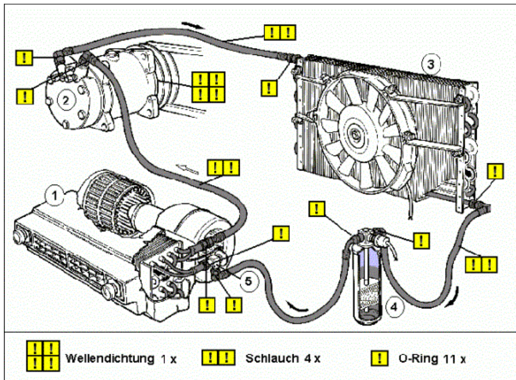
Abbildung 3.6: Der R 134a-Kältemittelkreislauf eines Pkw. Die Zahl der Ausrufezeichen (!) entspricht der Bedeutung einzelner Verlustquellen. Kältekreislauf: 1: Verdampfer, 2: Kompressor, 3: Kondensator, 4: Sammler/Trockner, 5: Expansionsventil. Aus: [WAECO 2000, modifiziert nach Schwarz 2001].
